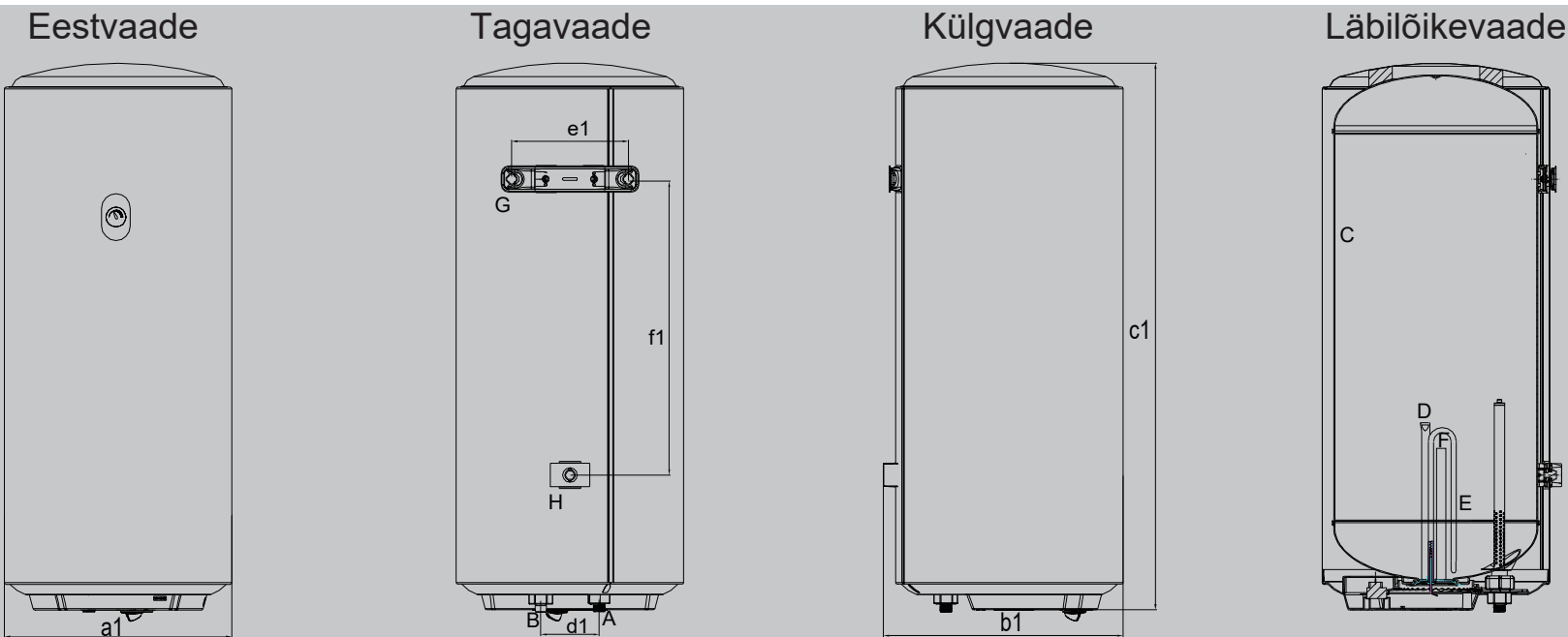
A: kuuma vee väljelaskeava B: külma vee sisselaskeava C: sisetuba D: temperatuuri mõõtetoru E: kütteelement F: magneesiumpulk G: seinakonks H: tugirühm
